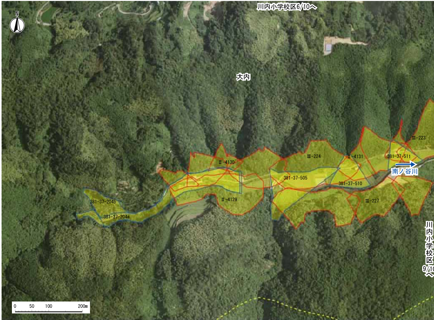
がけ崩れ
