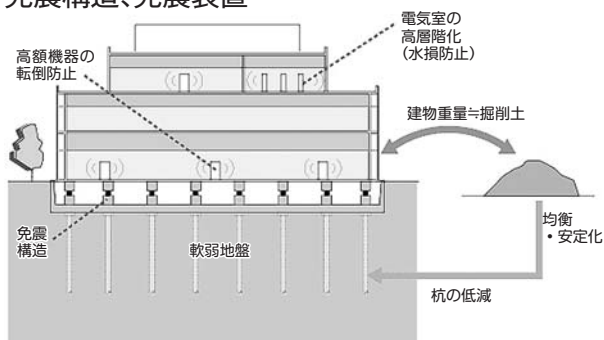
建物と医療機器及び医療機能を守る免震建物
